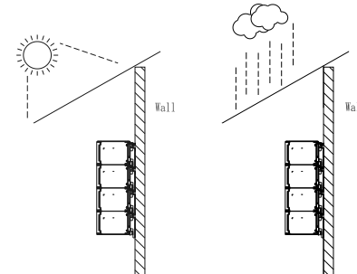
obr. 4.3: Přístřešky proti slunci a dešti
