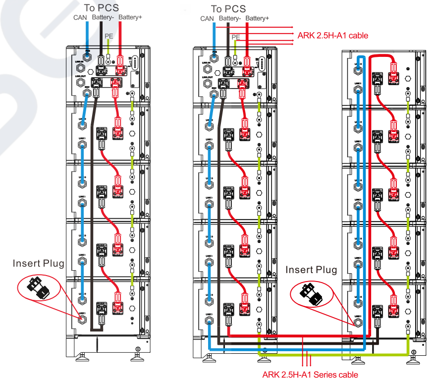
obr. 4.9: Instalace v jedné řadě
