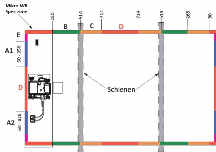
Abb. 1: Mit Schienenunterstützung
